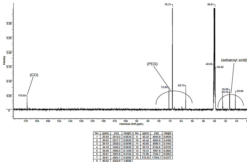
5-сурет. [ПЭГ]:[СК] негізіндегі сополимердің 13 C ЯМР-спектрі
