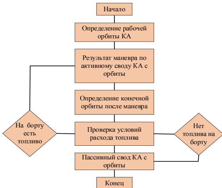
Рисунок 4 — Алгоритм расчета и моделирования начальных орбитальных параметров
