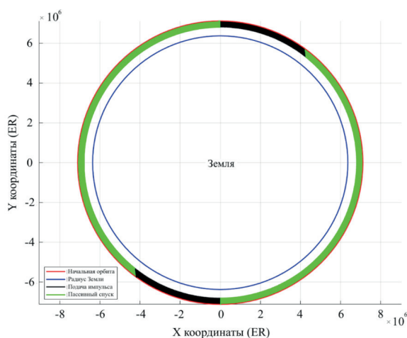
Рисунок 3 — График деорбитации КА при импульсивном торможении ДМТ
