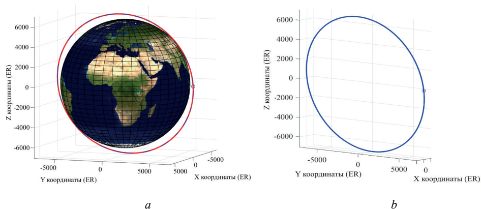
Рисунок 2 — Рабочая орбита КА и местоположение к началу расчета: a – с изображением Земли; б – без изображения Земли
